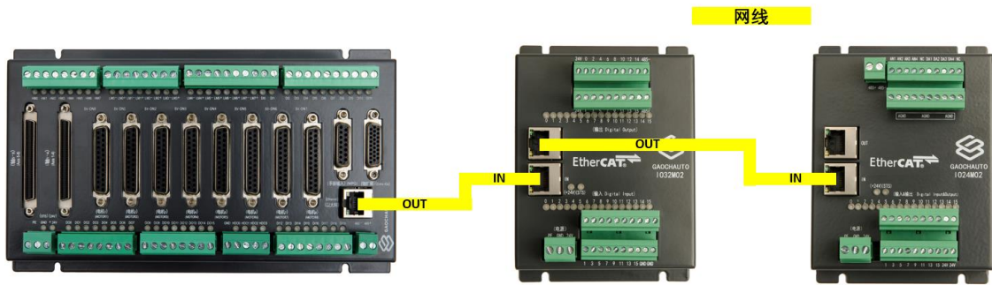
图 3.6.1 扩展模块接线示意图
