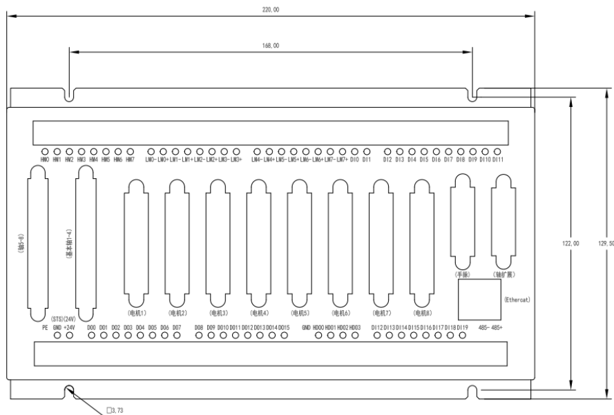
图 1.2.2 GC800A-PCIE 控制卡端子板外观及尺寸图
